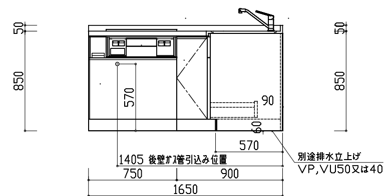
展開D図
