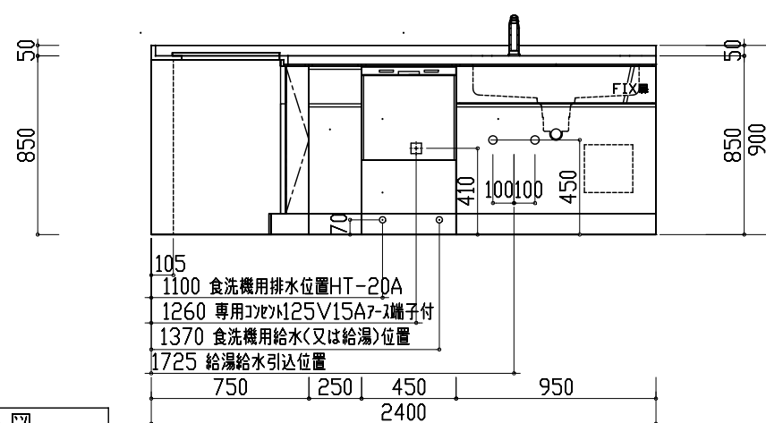
展開 A 図
