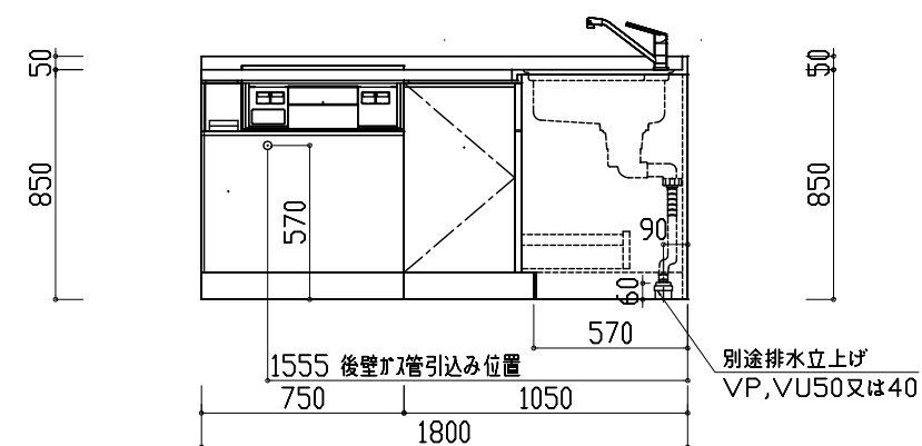
展開D図
