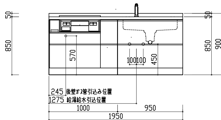
展開A図
