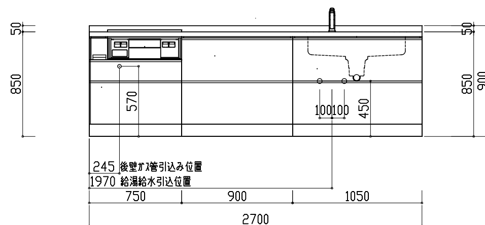
展開A図
