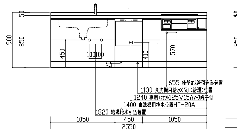
展開A図
