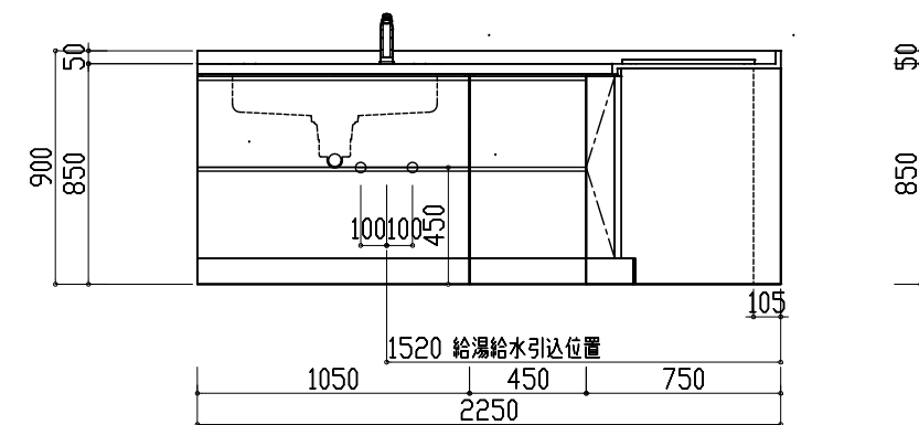
展開 A 図
